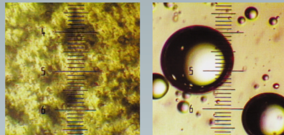
(1) Wasser in einer Hydraulikanlage (1) Water in the hydraulic system (1) L'eau dans une centrale hydraulique
