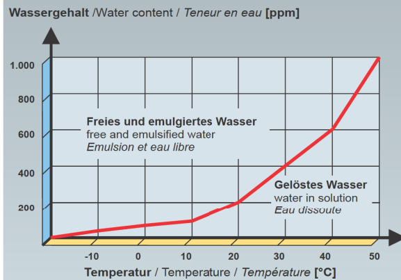
(2) Sättigungsgrenze für Wasser in einem Hydrauliköl (2) Saturation limit for water in a hydraulic oil (2) Seuil de saturation d'une huile
