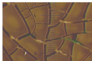
Fortgeschrittene Fluidalterung (Mikroskopaufnahme) Advanced fluid ageing (micro-photograph) Vieillessement avancé du fluide (Photo microscopique)
